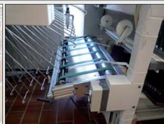
Bogenauslage mit Übergabeband zum Rütteltisch
